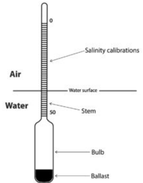
Fig. 2: Un hidrómetro de densidad.
