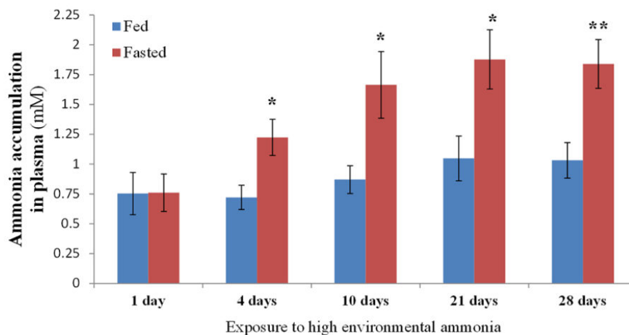
Fig. 2: Acumulación de amoníaco en la sangre de peces alimentados y privados de alimento después de la exposición a amoníaco ambiental alto durante 28 días. Los valores son media \pm S.E. Asterisco (*) denota diferencias significativas entre los peces alimentados y en ayunas (* P < 0.05 ; ** P < 0.01 ).
