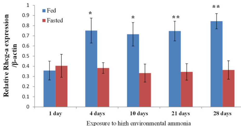
Fig. 4: Perfil de expresión de Rhcg-a en branquias de peces alimentados y privados de alimento después de la exposición a alto amoníaco ambiental durante 28 días. Los valores son media \pm S.E. Asterisco (*) denota diferencias significativas entre los peces alimentados y en ayunas (* P <0.05; ** P <0.01).
