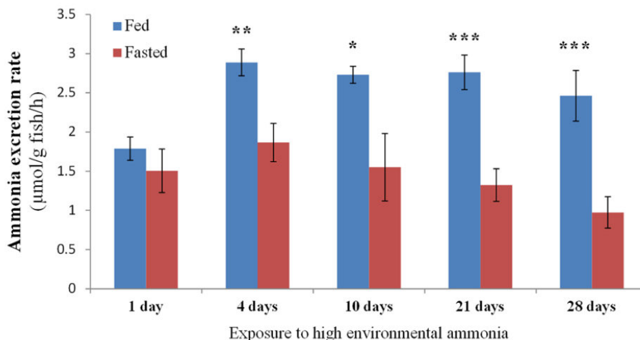
Fig. 3: Tasas de excreción de amoníaco por los peces alimentados y privados de alimento después de la exposición a alto amoníaco ambiental durante 28 días. Los valores son media \pm S.E. Asterisco (*) indica diferencias significativas entre los peces alimentados y en ayunas (* P < 0.05 ; ** P < 0.01 ; *** P < 0.001 ).
