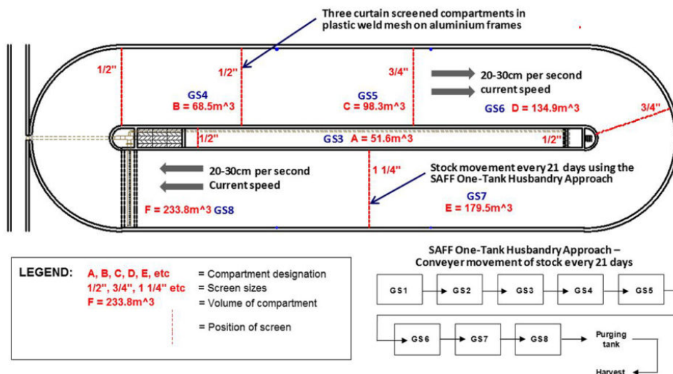
Fig. 2: Tanques de crecimiento de biofloc en Chambo Fisheries operados en un sistema de producción secuencial continuo (GS = Stanzas de crecimiento 3-8) aumentan la producción en un 150 por ciento sobre un sistema de producción por lotes.
