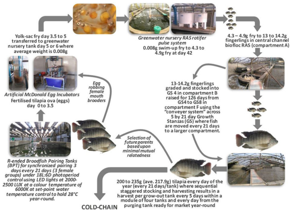
Fig. 1: Ciclo de vida de producción de tilapia de Shiranus ( Oreochromis shiranus ) de un módulo de cuatro tanques BFT produciendo hasta 400 toneladas por año de peces de 218 gramos durante todo el año.
