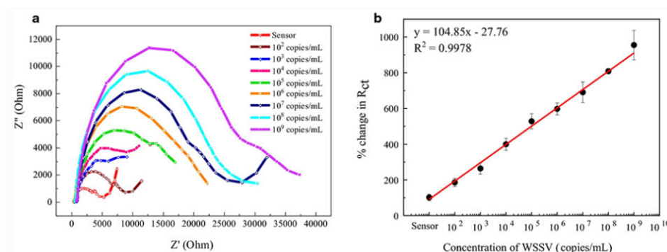
Fig. 1: Detección de WSSV utilizando el electrodo desechable. (a) Gráficos de resistencia para diferentes concentraciones de WSSV. Valores de eje en ohmios, unidades utilizadas para medir la resistencia eléctrica. (b) Curva de calibración de la impedancia correspondiente. El valor de resistencia de carga ( R_{ct} ) es una medida relevante para la electroquímica de corrosión y las reacciones electroquímicas. Cada detección se realizó tres veces y los datos se dan como promedio \pm DE ( n = 3 ).
